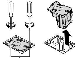
Befestigungsschrauben
