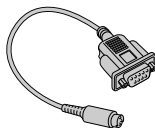
DIN-D-sub RS-232C 轉接頭 (5 57 / 64 " (15 cm)) <QCNWGA091 WJPZ>
