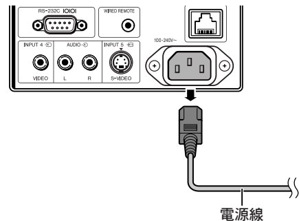
電源線
