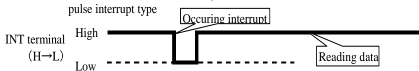
Fig.9 Interrupt output (pulse interrupt type )
