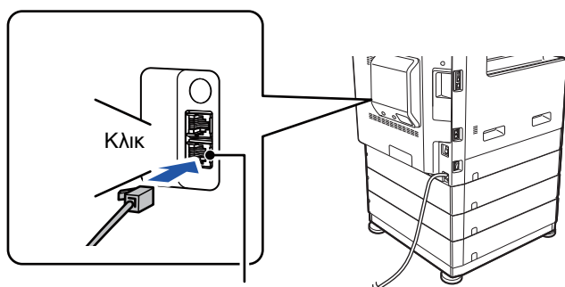
Υποδοχή τηλεφωνικής γραμμής (Line)
