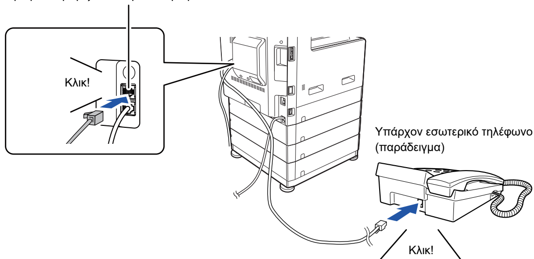
Τηλεφωνική πρίζα εσωτερικού τηλεφώνου
