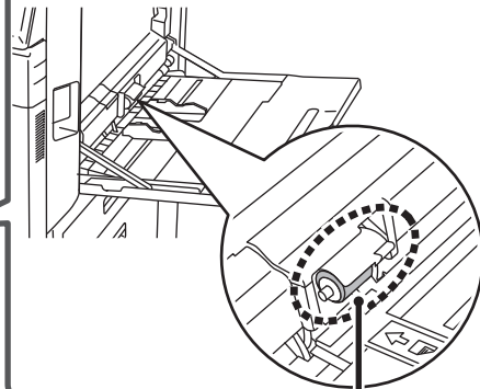
Podávací válec pomocného zásobníku
