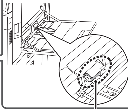
Doorvoerrol
