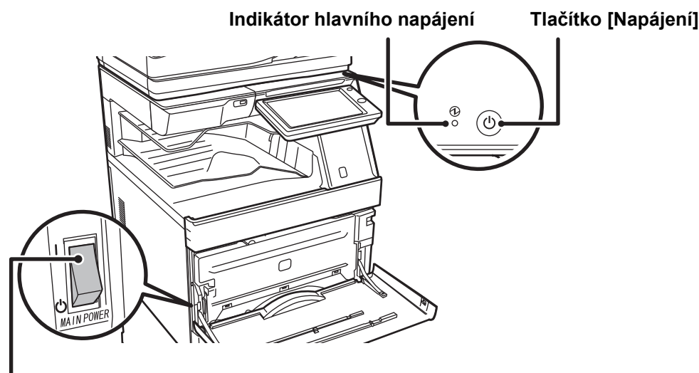
Hlavní vypínač
