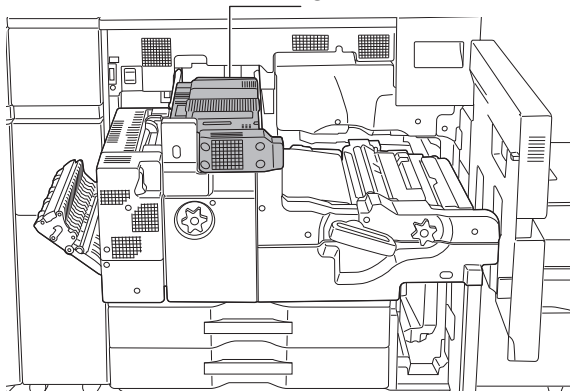
Unità fusore
