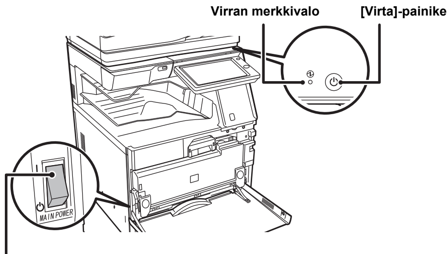
Päävirtakytkin
