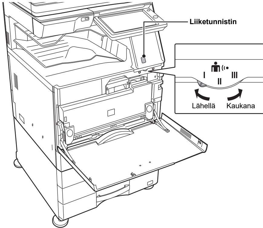
Havaintoalue
